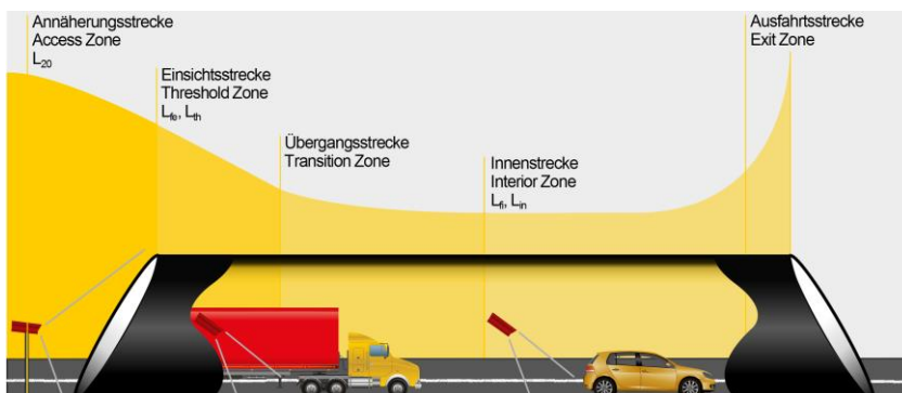
Gemessene Leuchtdichten im Tunnel und Installationsorte der Kameras
